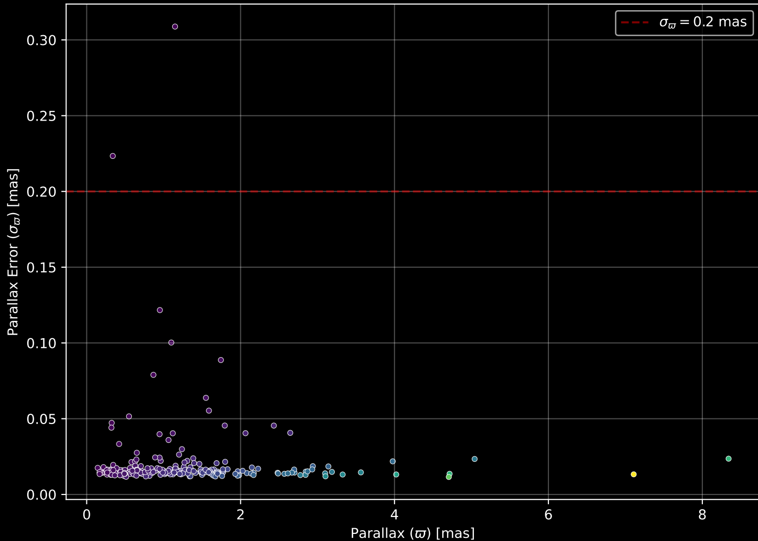
GALAH DR4 Field: [3857] Parallax Quality (n= 249)
