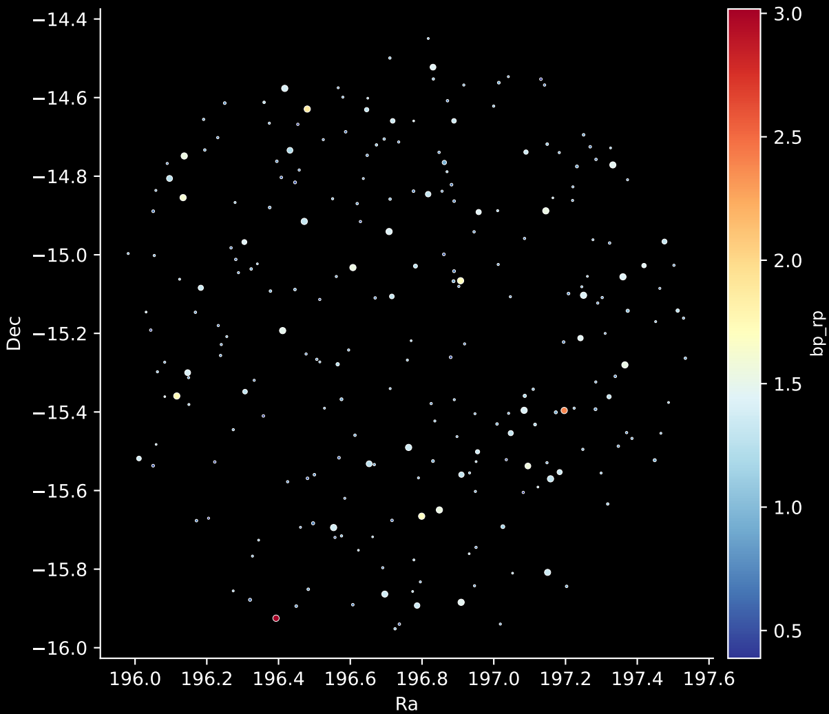
GALAH DR4 Field: [3857] Stars: 249
