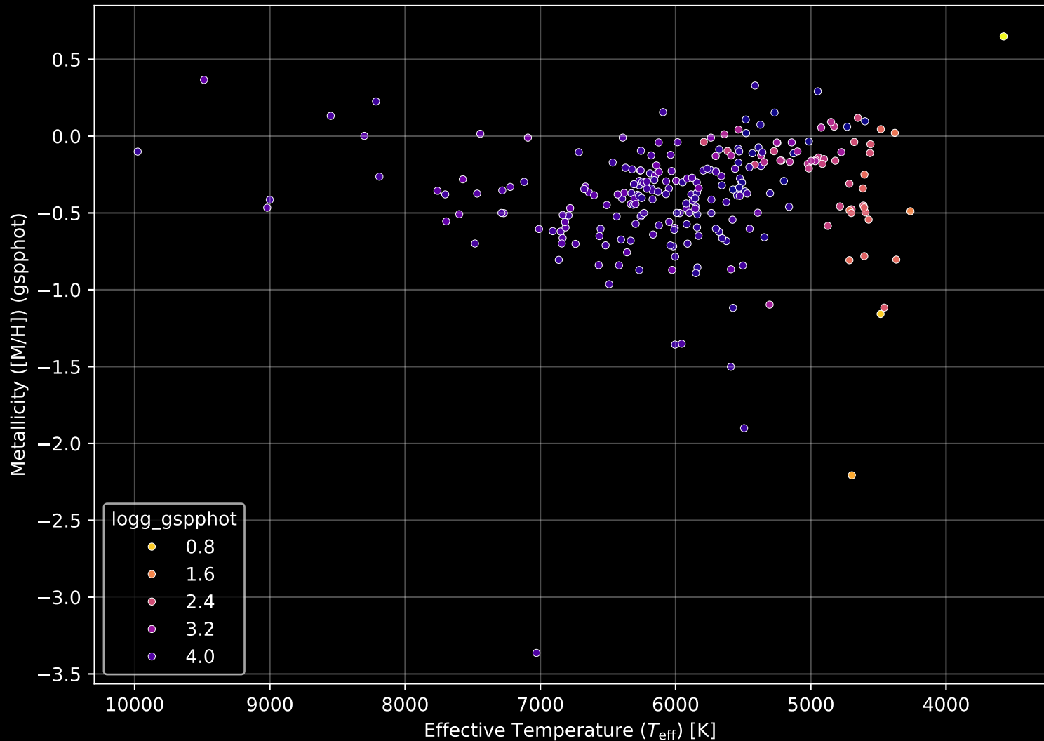
GALAH DR4 Field: [3857] Stellar Population Parameters (n= 249)
