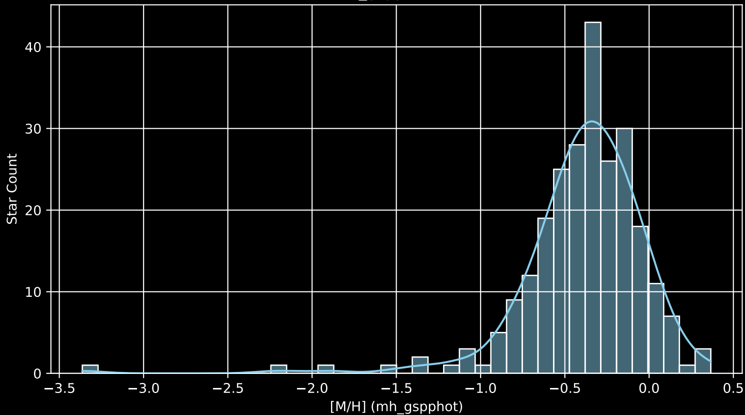
GALAH DR4 Field: [3857] [M/H] (mh_gspphot) (n= 248)
