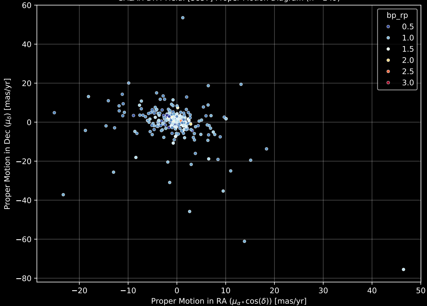
GALAH DR4 Field: [3857] Proper Motion Diagram (n= 249)
